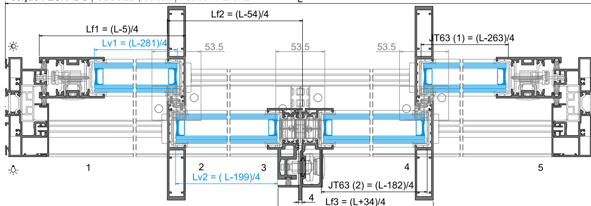
Posição FECHADO | CLOSED position | Position FERMÉ
