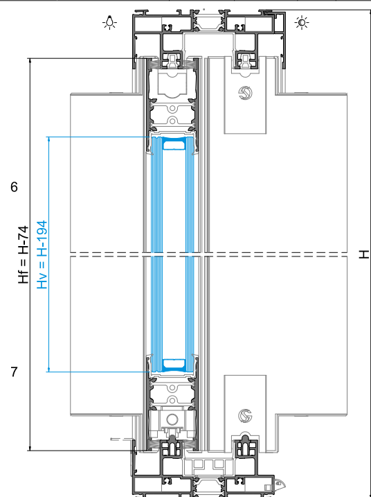
Posição ABERTO | OPEN position | Position OUVERT
