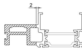
JT 74 Perfil ligação 2 folhas 2 Sashes connection profile Profilé pour connexion 2 vantaux
