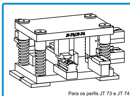
408068 CORTANTE JT - LIGAÇÃO 2 FOLHAS
