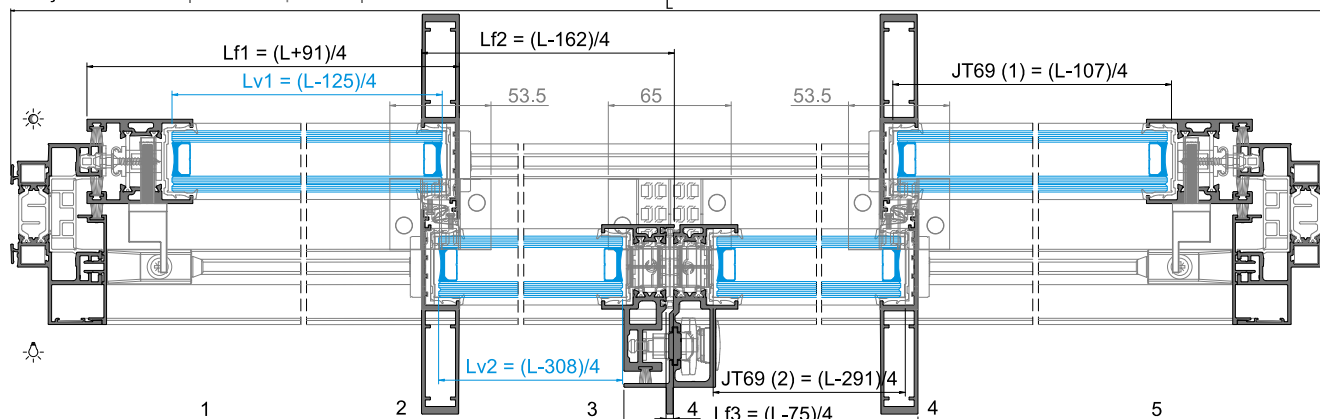
Posição FECHADO | CLOSED position | Position FERMÉ
