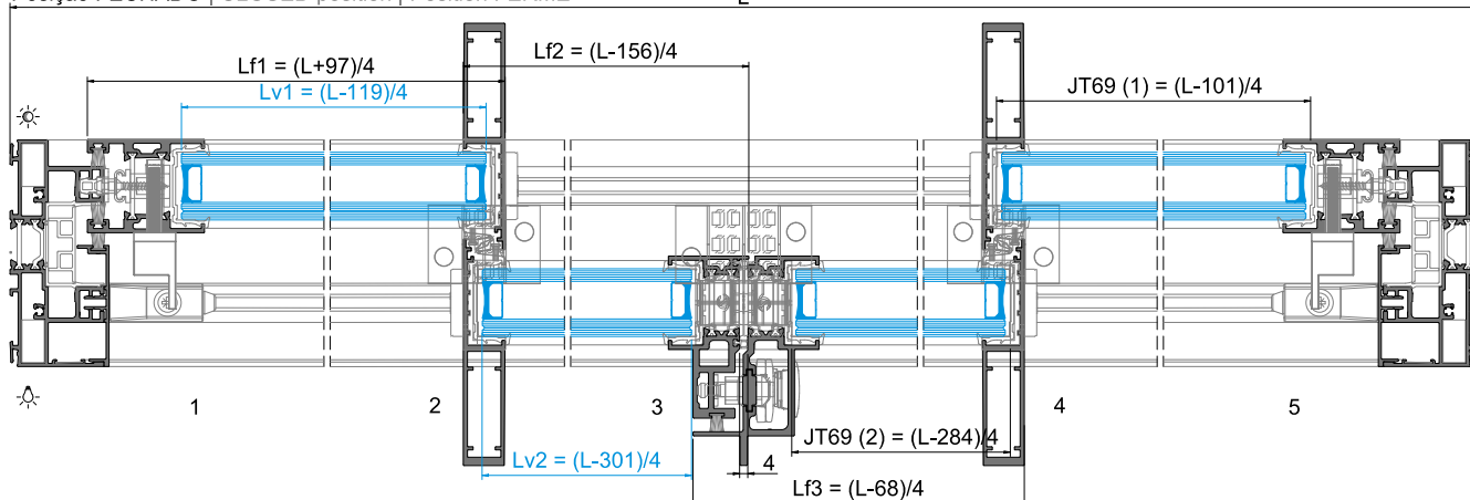
Posição FECHADO | CLOSED position | Position FERMÉ
