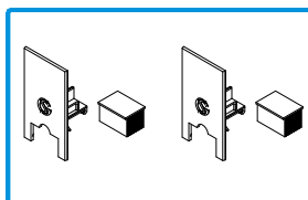
212339 CONJ. TAMPAS TOPOS CENTRAIS JT Nº1 Para os perfis JT 51, 52, 53 e 54 Material: Poliamida | Acabamento: Preto
