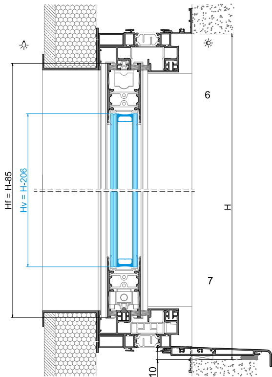
Posição FECHADO CLOSED position | Position FERMÉ
