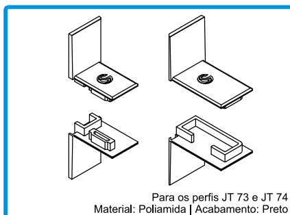
212408 CONJ. TAMPAS LIG. 2F JT73/JT74 JT-JT SLIM
