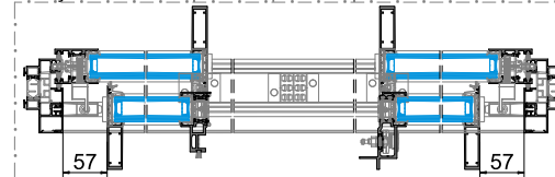
Posição ABERTO | OPEN position | Position OUVERT
