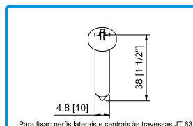
290262 PARAF. PAR 003 PK INOX PH 1 1/2x10 CQ Para fixar: perfis laterais e centrais às travessas JT 63, perfis JT 18 aos perfis JT12 e 22, os perfis SO47 e 48 Material: Inox | Acabamento: Inox
