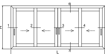
Posição FECHADO | CLOSED position | Position FERMÉ
