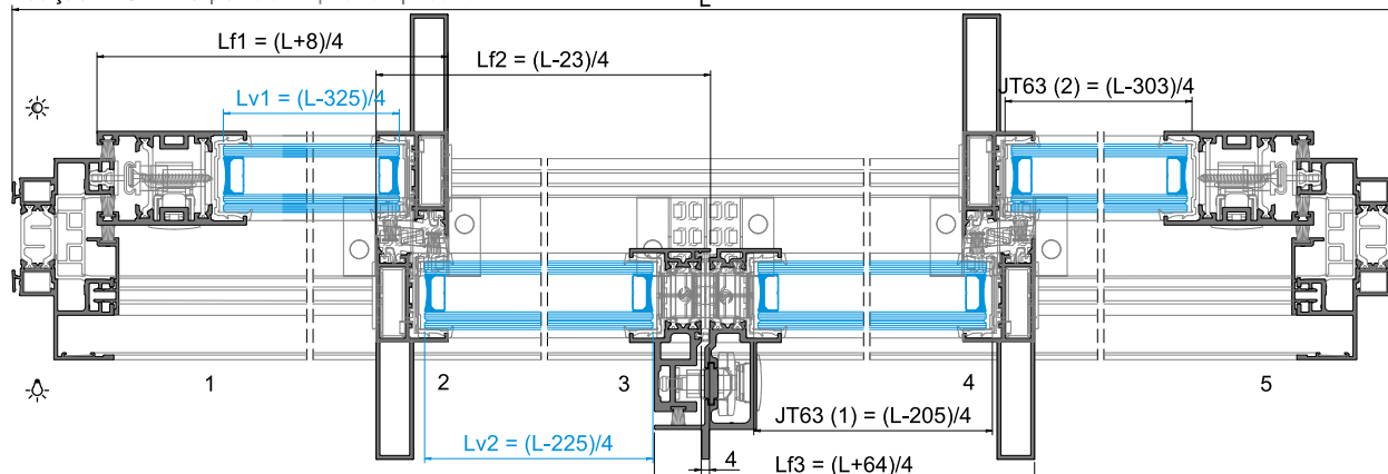
Posição FECHADO | CLOSED position | Position FERMÉ
