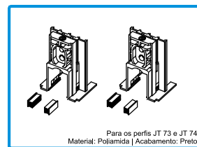
212407 CONJ. TOPOS LIG. 2F JT73/JT74 JT-JT SLIM
