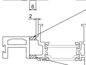
JT 74 Perfil ligação 2 folhas 2 Sashes connection profile Profilé pour connexion 2 vantaux
