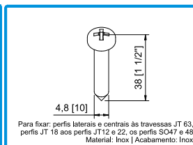
290262 PARAF. PAR 003 PK INOX PH 1 1/2x10 CQ
