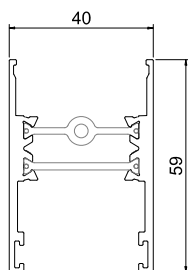
JT 69 Travessa inferior Lower transom | Traverse inférieur
