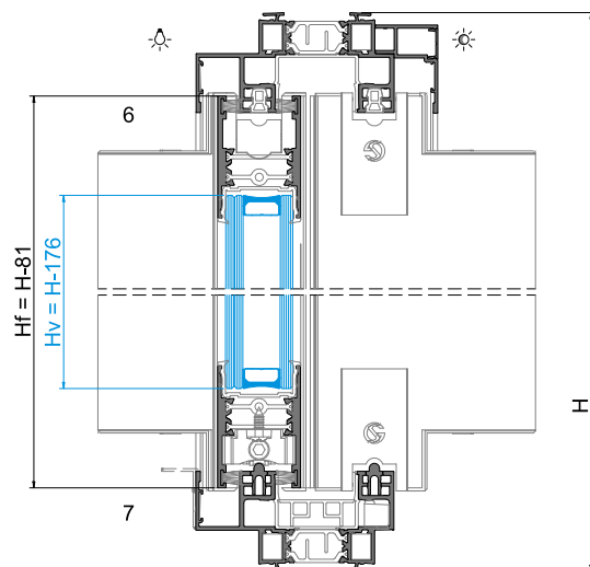
Posição ABERTO | OPEN position | Position OUVERT
