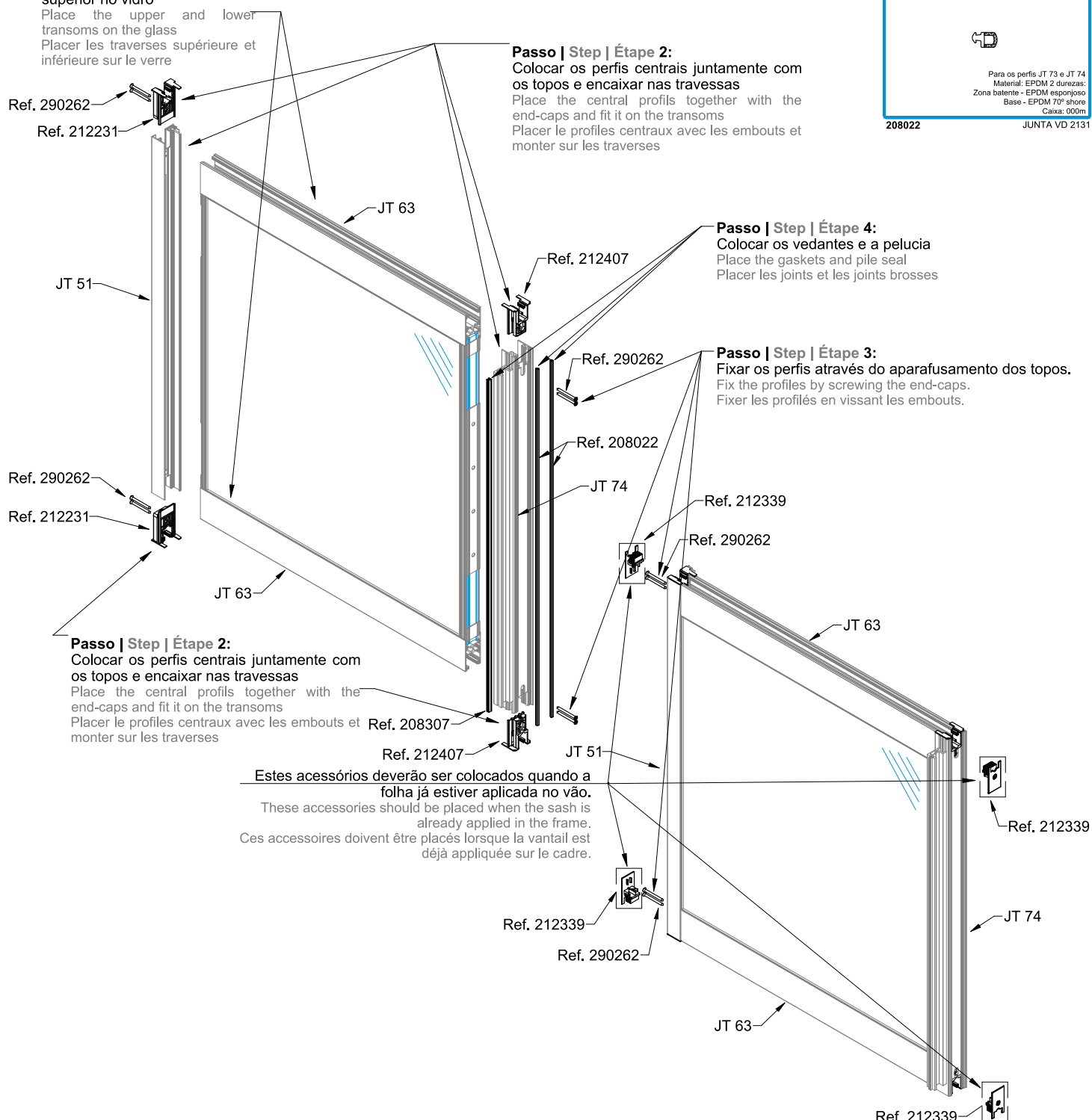
212407 CONJ. TOPOS LIG. 2F JT73/JT74 JT-JT SLIM Para os perfis JT 73 e JT 74 Material: Poliamida | Acabamento: Preto
