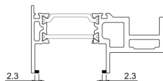
JT 74 Perfil ligação 2 folhas 2 Sashes connection profile Profilé pour connexion 2 vantaux
