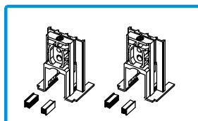
212407 CONJ. TOPOS LIG. 2F JT73/JT74 JT-JT SLIM Para os perfis JT 73 e JT 74 Material: Poliamida | Acabamento: Preto
