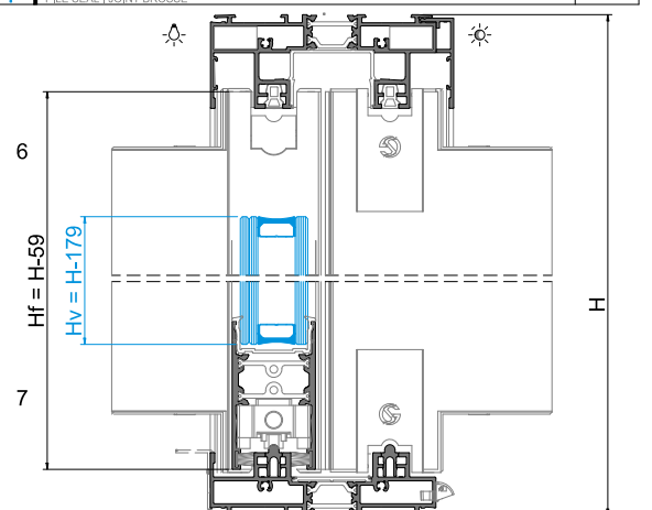
Posição ABERTO | OPEN position | Position OUVERT
