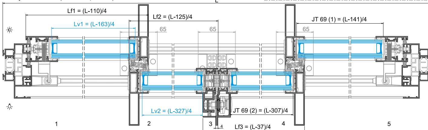
Posição FECHADO | CLOSED position | Position FERMÉ
