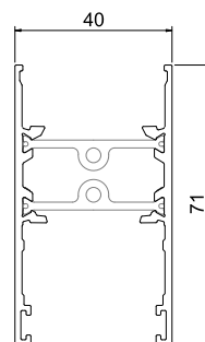
JT 63 Travessa inferior Lower transom | Traverse inférieur
