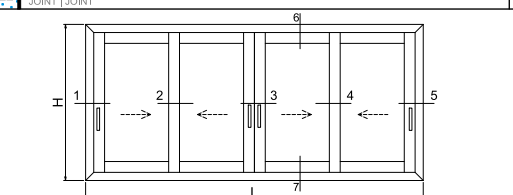
Posição FECHADO | CLOSED position | Position FERMÉ
