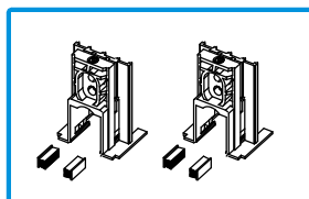
212407 CONJ. TOPOS LIG. 2F JT73/JT74 JT-JT SLIM Para os perfis JT 73 e JT 74 Material: Poliamida | Acabamento: Preto
