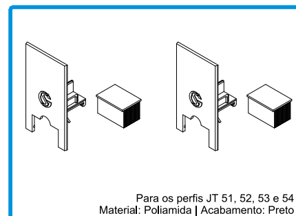
212339 CONJ. TAMPAS TOPOS CENTRAIS JT Nº1
