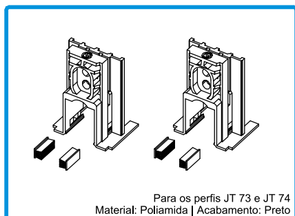
212407 CONJ. TOPOS LIG. 2F JT73/JT74 JT-JT SLIM
