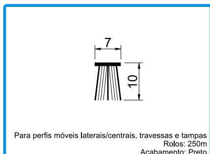
208307 PELÚCIA 7x10 TRI-FIN Preto
