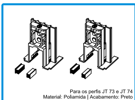
212407 CONJ. TOPOS LIG. 2F JT73/JT74 JT-JT SLIM
