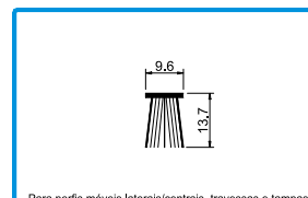
208306 PELÚCIA 7x10 TRI-FIN Cinza 208307 PELÚCIA 7x10 TRI-FIN Preto Para perfis móveis laterais/centrais, travessas e tampas Rolos: 250m Acabamentos: Preto ou Cinza
