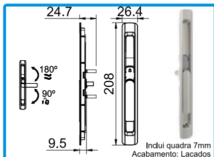
201083 FECHO DE EMBUTIR 180°
