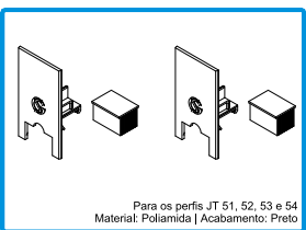
212339 CONJ. TAMPAS TOPOS CENTRAIS JT N°1
