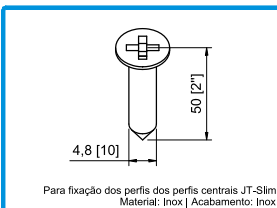
290091 PARAFUSO DIN7982 PH 4,8x50 A2
