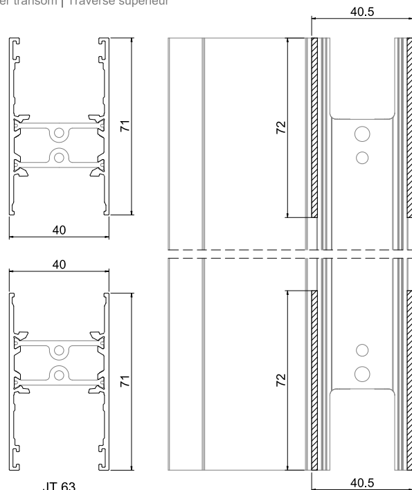
JT 63 Travessa inferior Lower transom | Traverse inférieur
