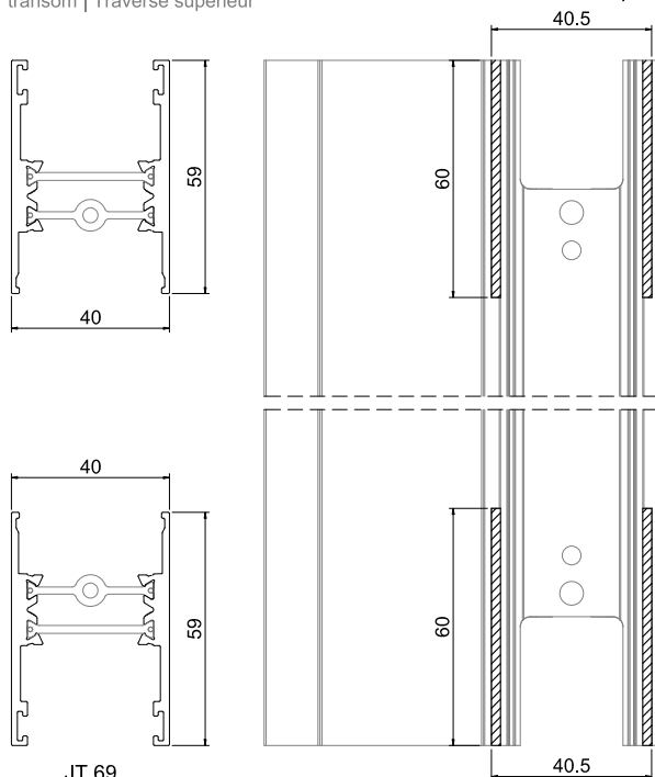
JT 69 Travessa inferior Lower transom | Traverse inférieur
