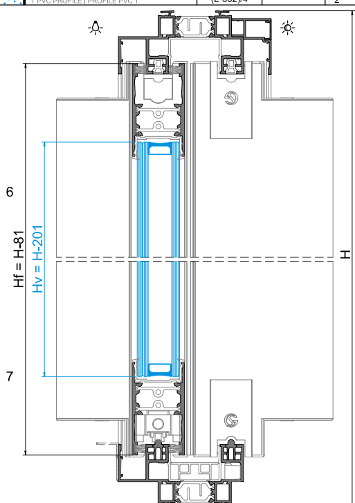
Posição ABERTO | OPEN position | Position OUVERT
