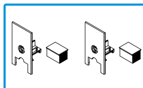
212339 CONJ. TAMPAS TOPOS CENTRAIS JT Nº1 Para os perfis JT 51, 52, 53 e 54 Material: Poliamida | Acabamento: Preto
