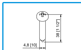
290262 PARAF. PAR 003 PK INOX PH 1 1/2x10 CQ Para fixar: perfis laterais e centrais às travessas JT 63, perfis JT 18 aos perfis JT12 e 22, os perfis SO47 e 48 Material: Inox | Acabamento: Inox
