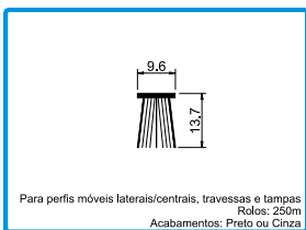
208306 208307 PELÚCIA 7x10 TRI-FIN Cinza PELÚCIA 7x10 TRI-FIN Preto
