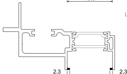
JT 73 Perfil ligação 2 folhas reforçado 2 Sashes connection reinforced profile Profilé pour connexion 2 ventaux renforcé
