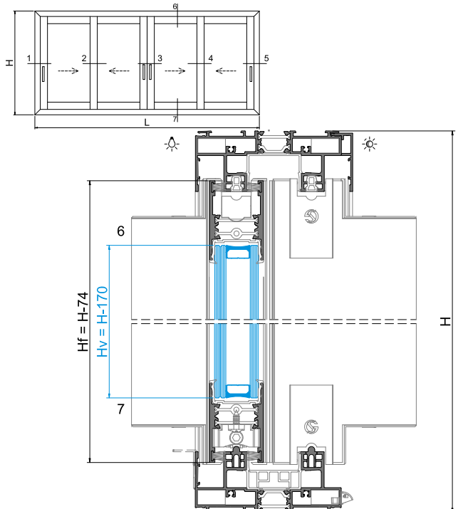
Posição ABERTO | OPEN position | Position OUVERT
