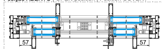
Posição ABERTO | OPEN position | Position OUVERT
