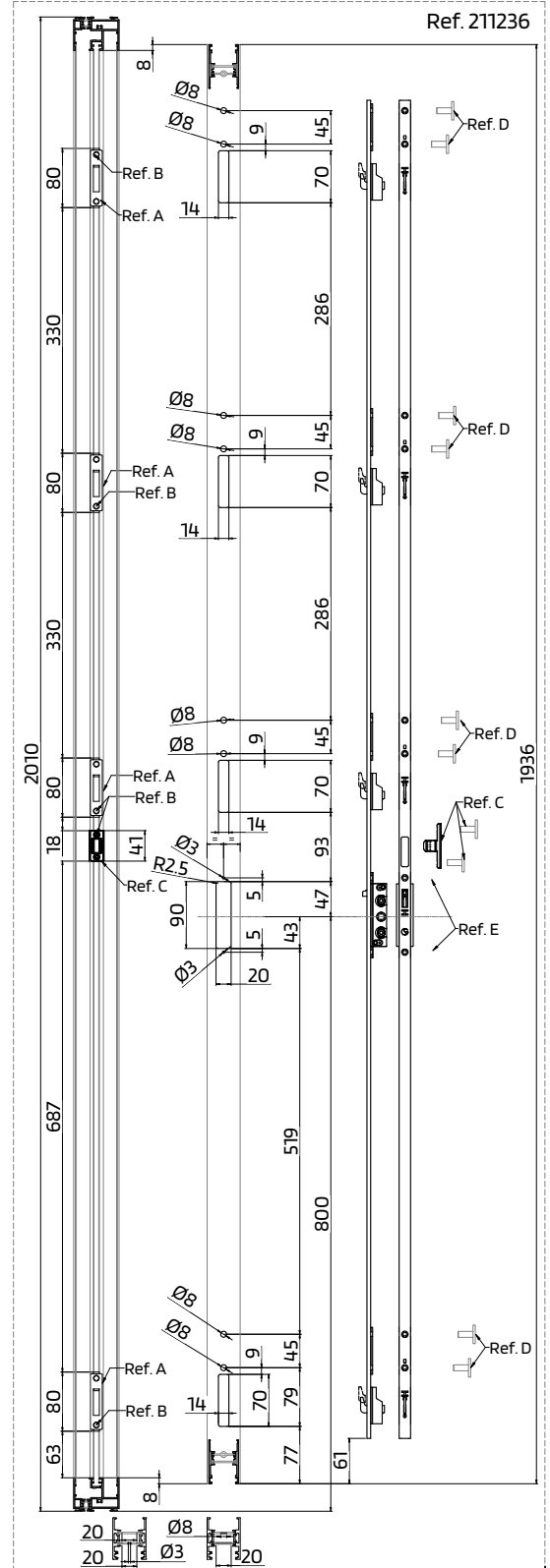
Para fixação das ferragens multiponto 212373 CONJ. FIXAÇÃO JT-SLIM
