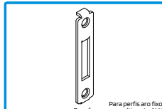
Para perfis aro fixo Para ferragens multiponto ALU Material: Inox | Acabamento: Inox 202330 CONTRA-FECHO ALU
