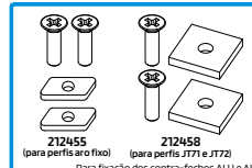
Para perfis aro fixo (para perfis JT71 e JT72) Para fixação dos contra-fechos ALU e AL Acabamentos: Inox (refs 212455/58) e Preto (ref 212455) 212455 CONJ. FIX. C-FECHO AL MULTIP. JT 212458 CONJ. FIX. C-FECHO 2F/90° JT
