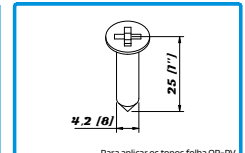
Para aplicar os topos folha GR-PV Material: Inox | Acabamento: Inox 290078 PARAF. DIN7982 PH 4.2x25 INOX A2
