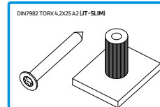
Para fixação das ferragens multiponto 212373 CONJ. FIXAÇÃO JT-SLIM
