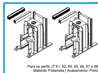
212199 CONJ. TOPOS LAT. JT Nº1
