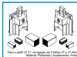
212295 CONJ. TOPOS LIGAÇÃO 2 FOLHAS JT-JT SLIM
