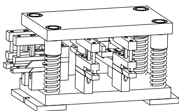
408175 CORTANTE ESQUADROS OS N° 2
