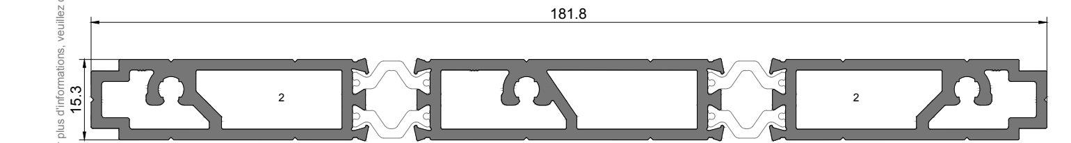
SO 93 Pré-aro 3-rail 3-rail Pre-frame profile | Profilé pré-châssis 3-rail
