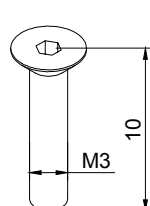
290016 PARAFUSO FIXAÇÃO DE TOPOS
