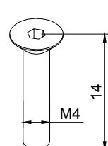
290473 PARAFUSO DIN7991 M4X14 INOX A2
