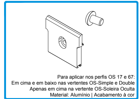
210096 TOPO CENTRAL INVERTIDO N° 4 OS-V2
