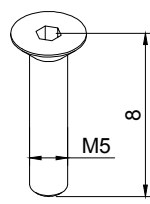
290099 PARAF. DIN7991 M5X8 INOX A2
