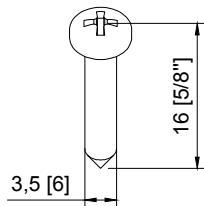
290729 PARAF PKI PH 5/8x6 CQ
