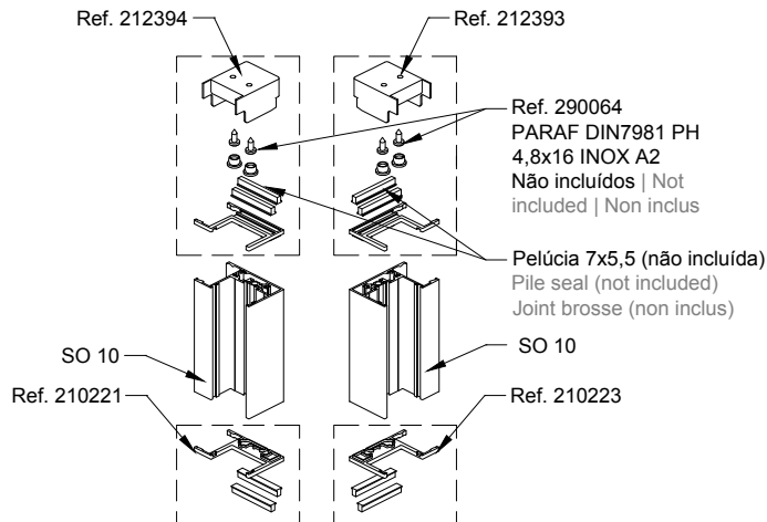
212394 CONJ. TOP. SUP/INF CANTO FIXO SO 10 ESQ
