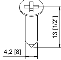
290061 PARAF. DIN7982 PH 4,2x13 INOX A2
