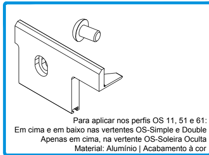
210094 TOPO CENTRAL N°2 OS V2 ESQUERDO
