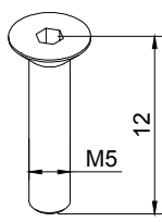
290059 PARAFUSO DIN7991 M5x12 INOX A2
