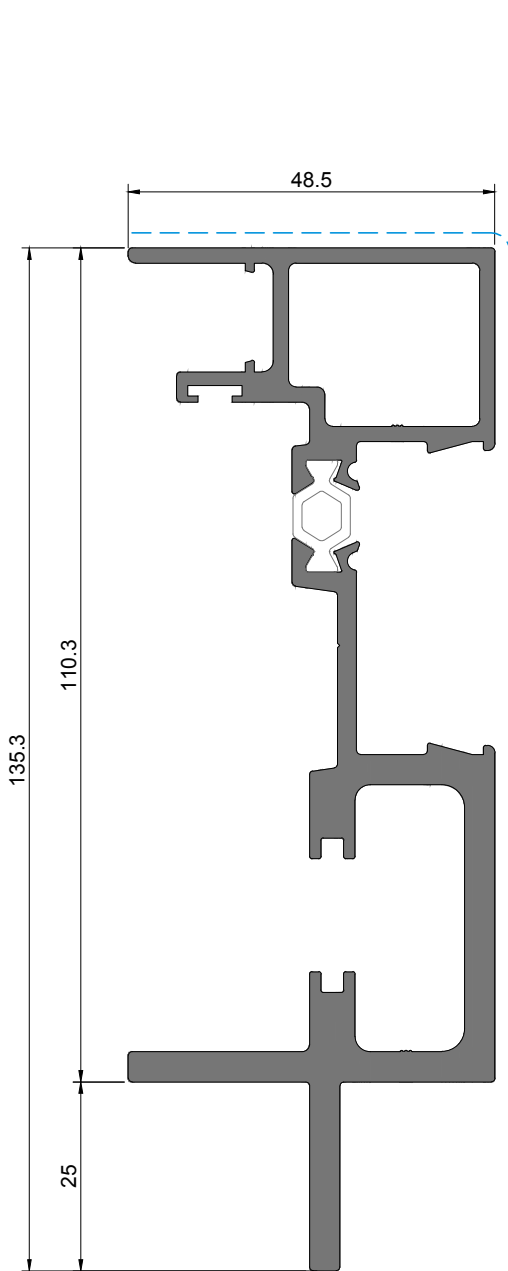
SO 39 Perfil ligação 2 folhas 2 Sashes connection profile Profilé pour connexion 2 vantaux
