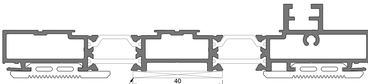
JT 27 Ombreira 90° 3rail 3rail 90° jamb | Jambage 90° 3rail
