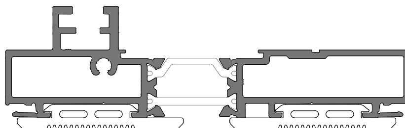
JT 19 Ombreira 90° 2rail 2rail 90° jamb | Jambage 90° 2rail
