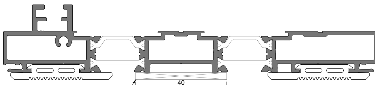
JT 29 Ombreira 90° 3rail 3rail 90° jamb | Jambage 90° 3rail
