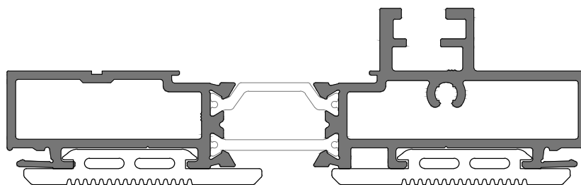
JT 17 Ombreira 90° 2rail 2rail 90° jamb | Jambage 90° 2rail
