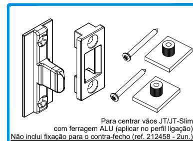
212291 CONJ. CENTRADOR P/ FERR. ALU PERFIL LIG.
