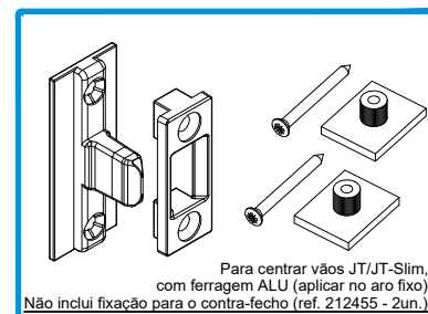
212289 CONJ. CENTRADOR P/ FERR. ALU
