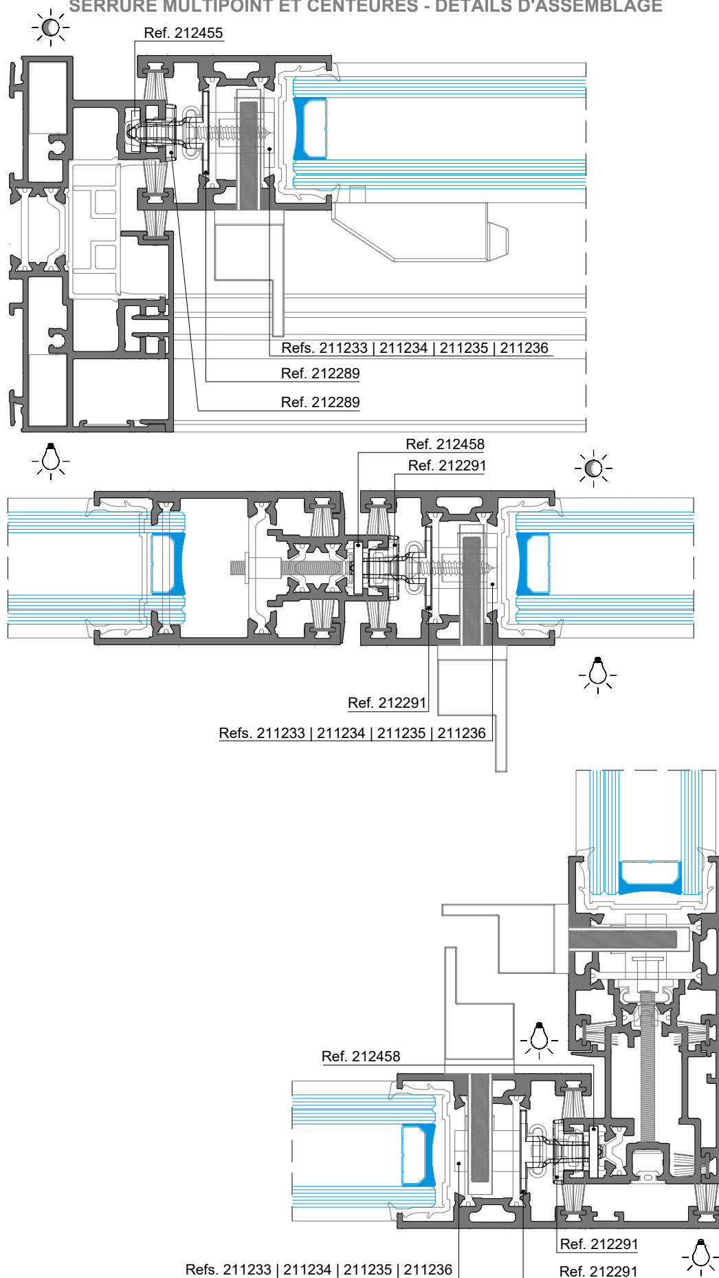
212289 CONJ. CENTRADOR P/ FERR. ALU
