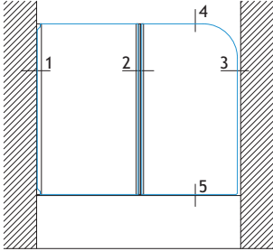
SEM PERFIL DE PAREDE RB 14 WITHOUT WALL PROFILE RB 14 SANS PROFIL DE MUR RB 14
