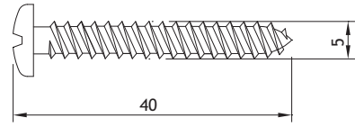
290106 PARAFUSO AGL CQ INOX A2 5x40 RB
