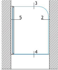
COM PERFIL DE PAREDE RB 14 WITH WALL PROFILE RB 14 AVEC PROFIL DE MUR RB 14
