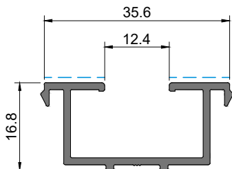
JL 24 Perfil redutor Slot reduction profile | Profilé de réduction
