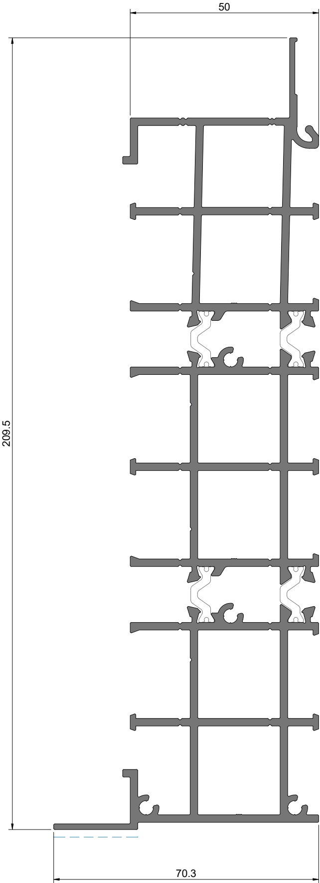
VO 23 Soleira alta 3-rail para caleira 3-rail high Sill for drainage gutter | Seuil haut 3-rail pour gouttière de sol
