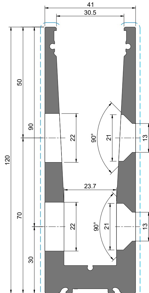
AV 15 Com furações laterais With lateral milling Avec fraisage latéral
