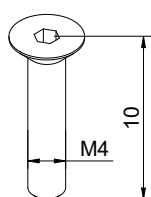
290138 PARAFUSO DIN7991 M4X10 INOX A2
