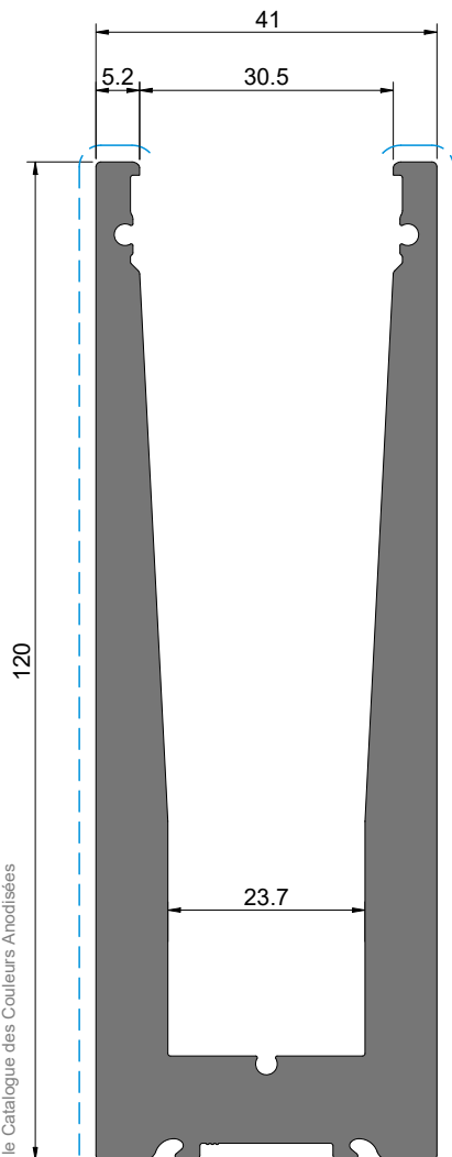
AV 01 Sem furações Without milling Sans fraisage
