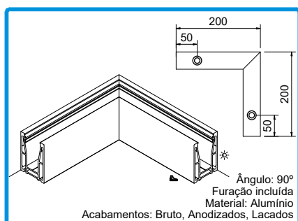
213033 CANTO 90° INTERIOR AV 27
