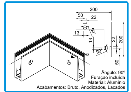
213022 CANTO 90° INTERIOR AV14
