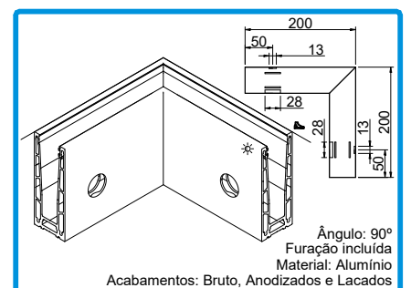
213037 CANTO 90° EXTERIOR AV 25
