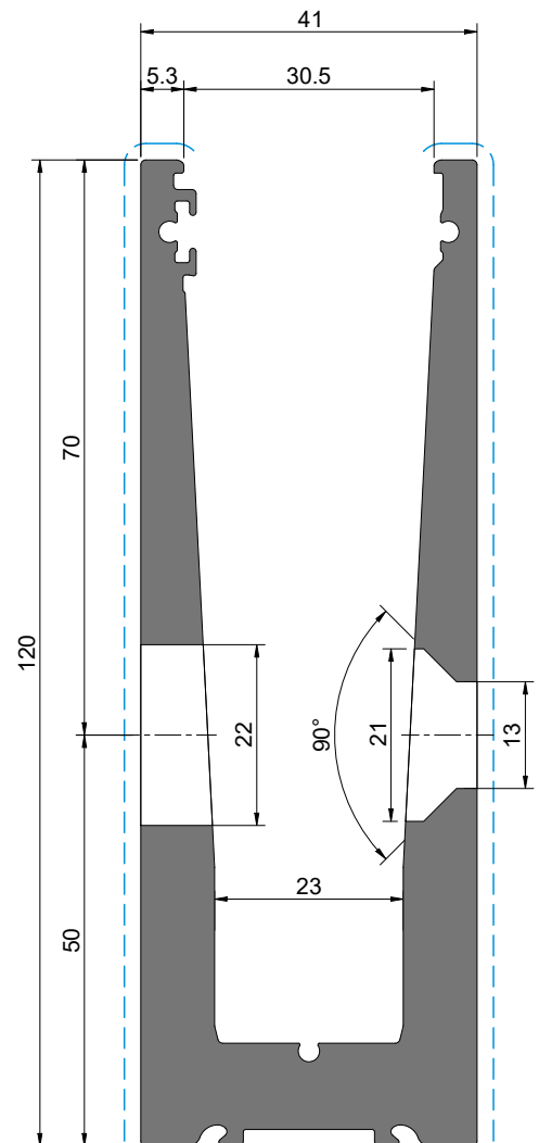
AV 14 Com furações laterais With lateral milling Avec fraisage latéral
