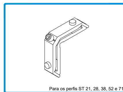
204901 ESQUADRO 18-1112-C
