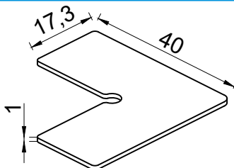
213018 CANTO DE ALINHAMENTO OS Nº2
