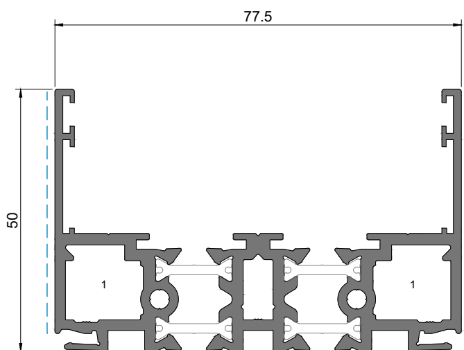
SO 34 Soleira 1-rail Sill | Seuil 1-rail
