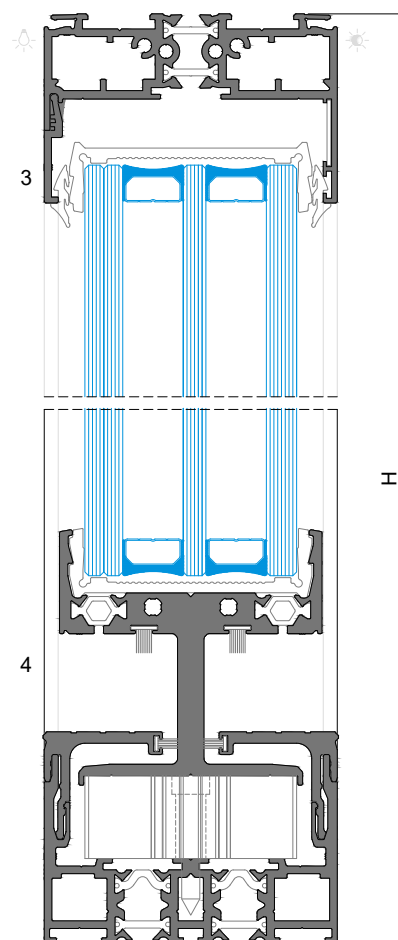
PERFIL | PROFILE | PROFILÉ - OS 38
