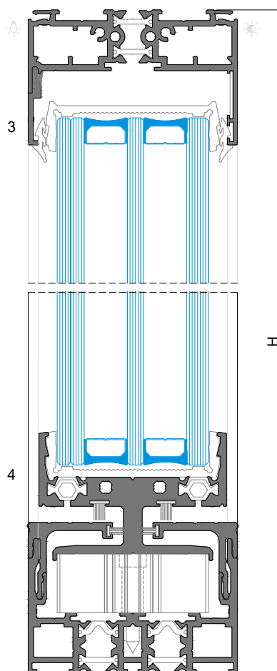
PERFIL | PROFILE | PROFILÉ - OS 28
