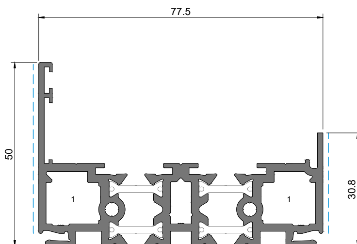
VO 34 Soleira 1-rail Sill | Seuil 1-rail
