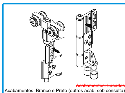
207282 ROLAMENTO E DOBRADIÇA HARMÔNIO INF./SUP.
