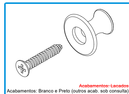
299936 APLIQUE FIXADOR
