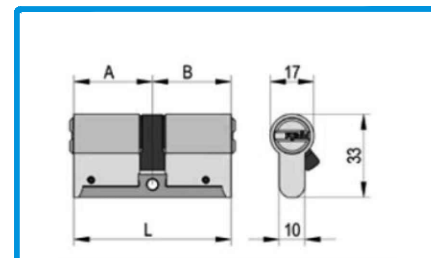
207436 CILINDRO ALTA SEGURANÇA 30/30
