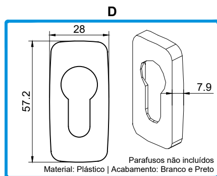
220190 ESPELHO PARA SEGURANÇA 874.801
