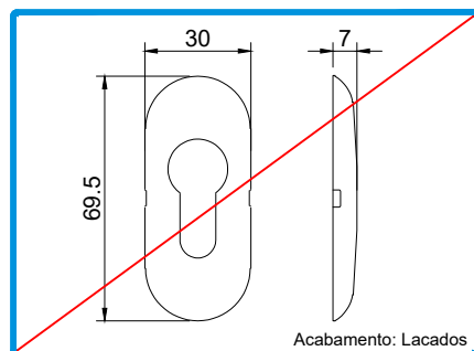
220251 ESPELHO P/SEGredo 3500
