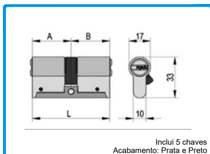
207407 CILINDRO ALTA SEGURANÇA 45/45
