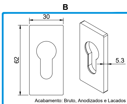
220197 ESPELHO ALUMÍNIO 30MM P/ SEGREDO
