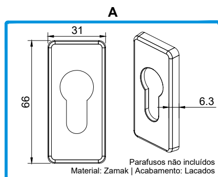
220198 ESPELHO DELTA P/ SEGREDO
