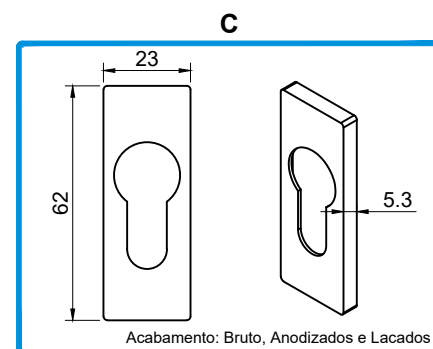
220196 ESPELHO ALUMÍNIO 23MM P/ SEGREDO
