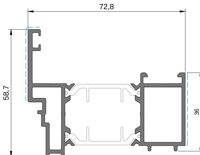
ST 94 Perfil para fechadura Lock profile | Profilé pour serrure
