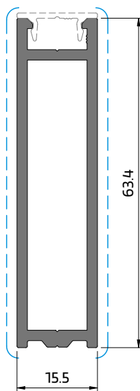
SO 67 Perfil de reforço Reinforcement profile | Profilé de reinforcement
