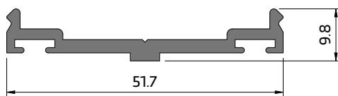
FC 04 Suporte para capa Cap bracket | Porte-capot
