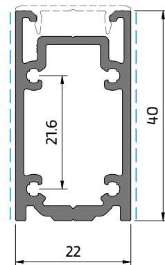
JE 35 Perfil de reforço Reinforcement profile | Profilé de reinforcement
